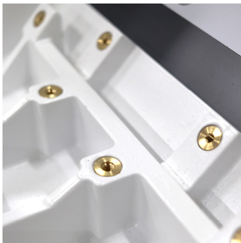
Posage d'inserts
